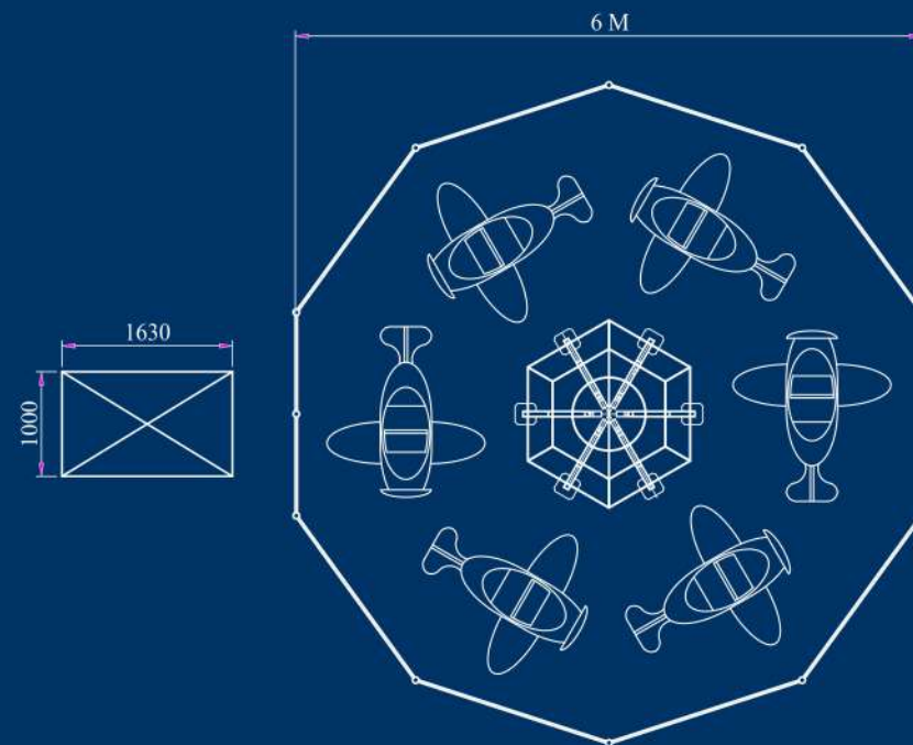
ПЛАН
